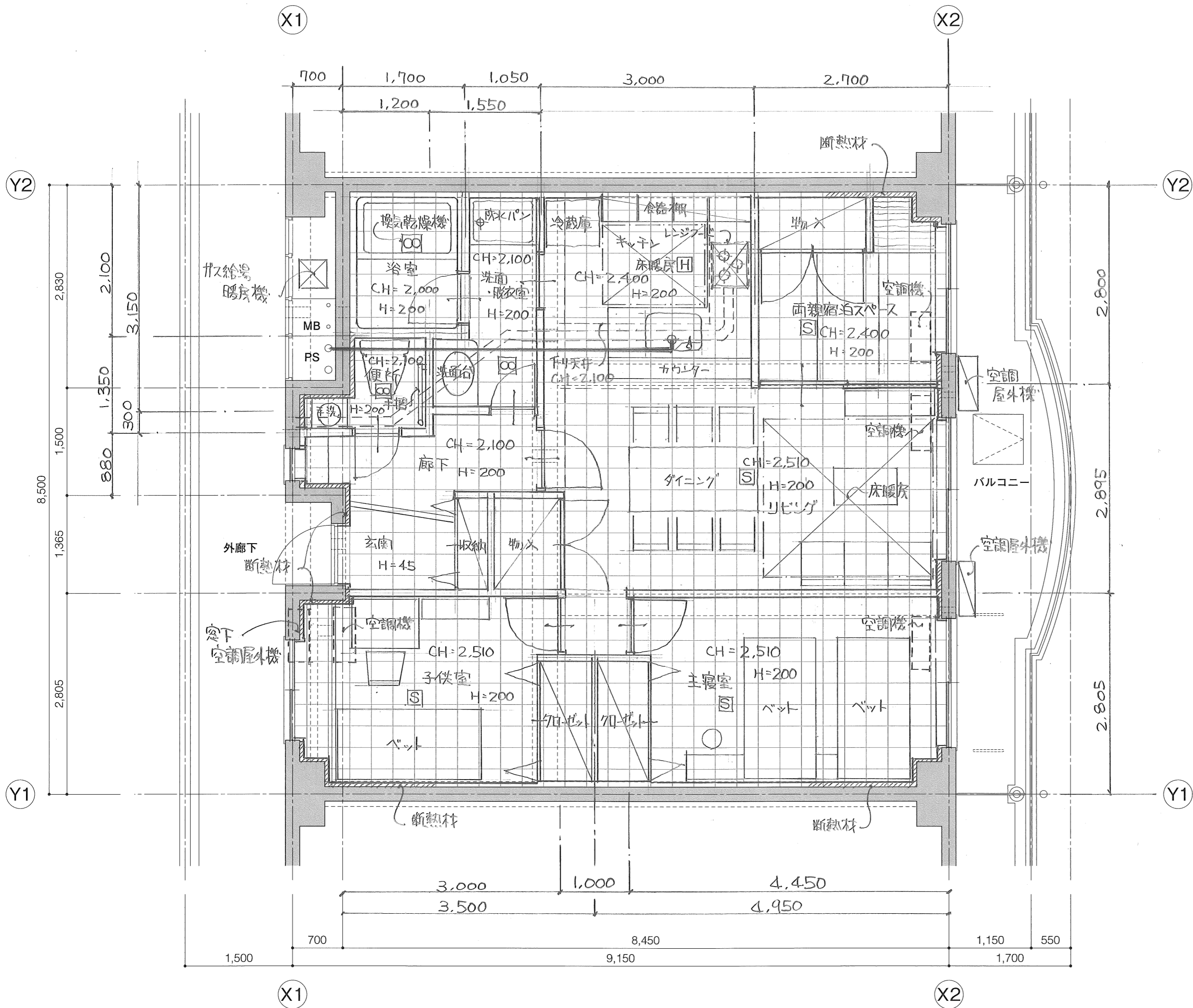
平面図 (縮尺: 1/50)
