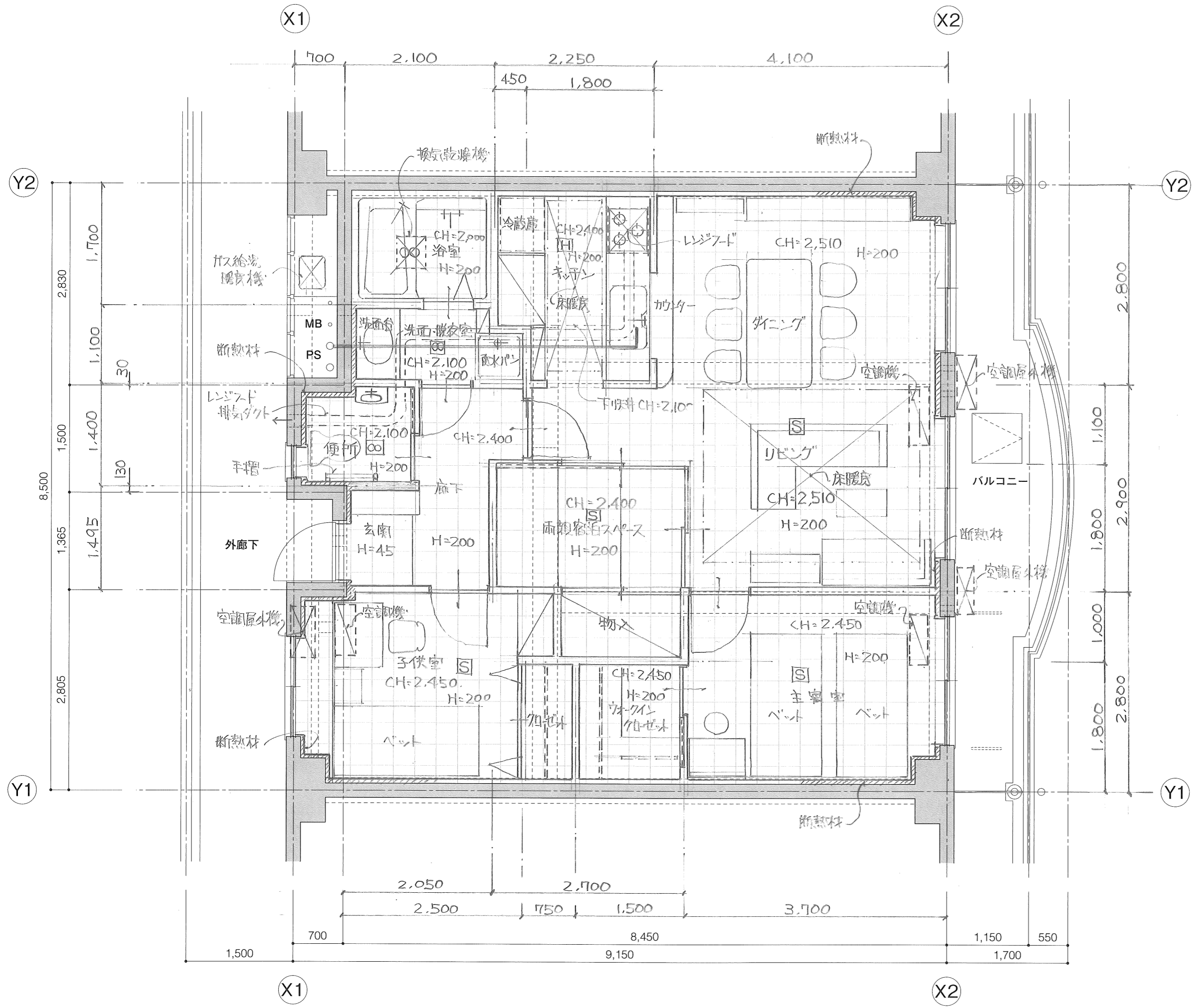
平面図 (縮尺: 1/50)
