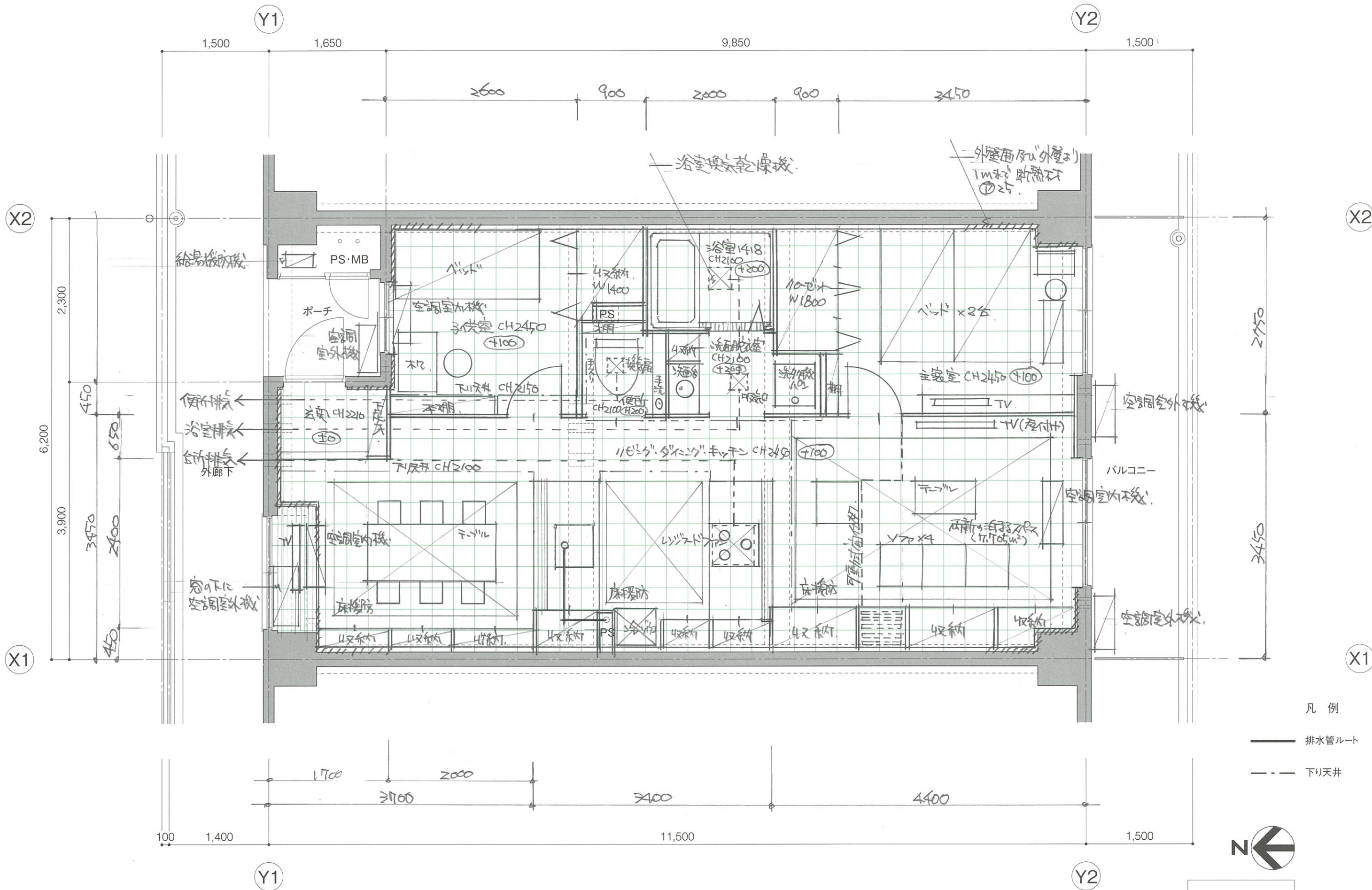
(2) 平面図 (縮尺: 1/50)
