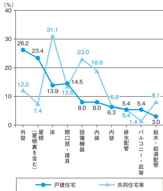
図2-30 住宅形式別に見る主な不具合部位の割合 (リフォーム) ※複数カウント
