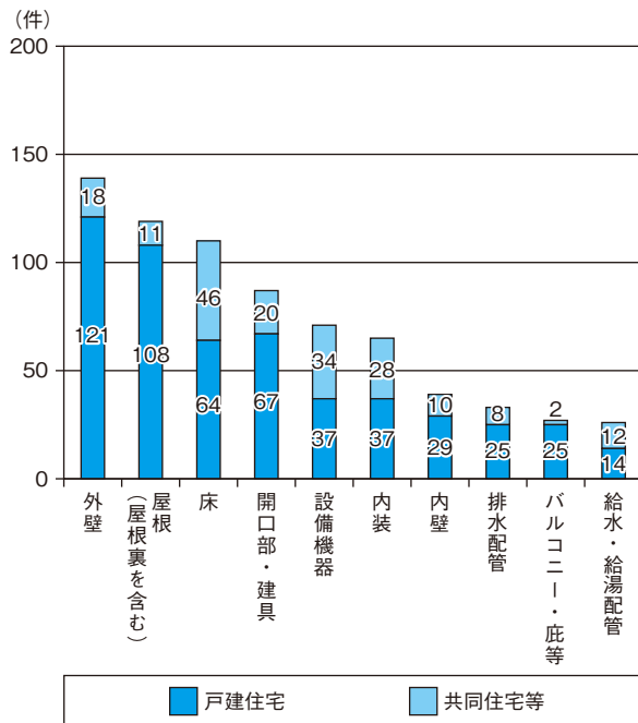
図2-29 住宅形式別に見る主な不具合部位 (リフォーム) ※複数カウント
